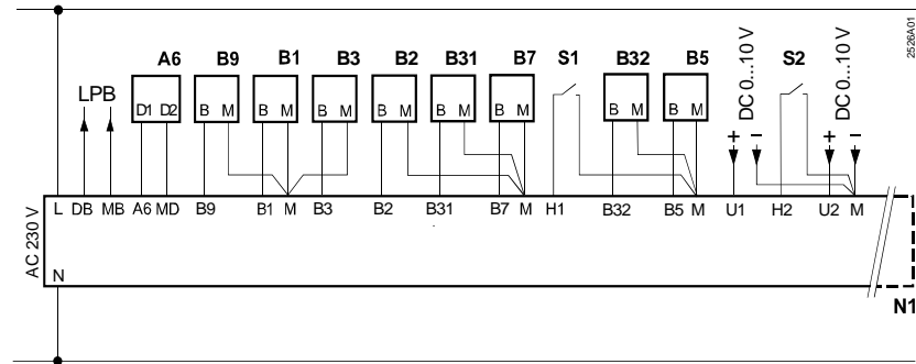
Grundsätzliche Anschlüsse für Anlagen mit externen Wärmebedarfssignalen
