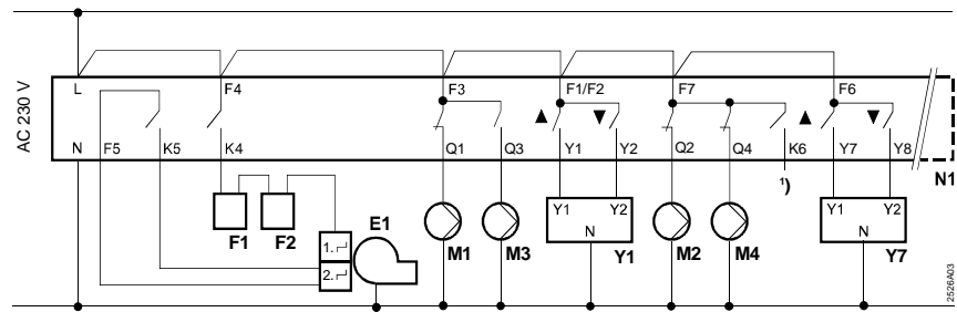
Grundsätzliche Anschlüsse für Anlagen mit zweistufigem Brenner
