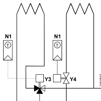
Zonenventil
